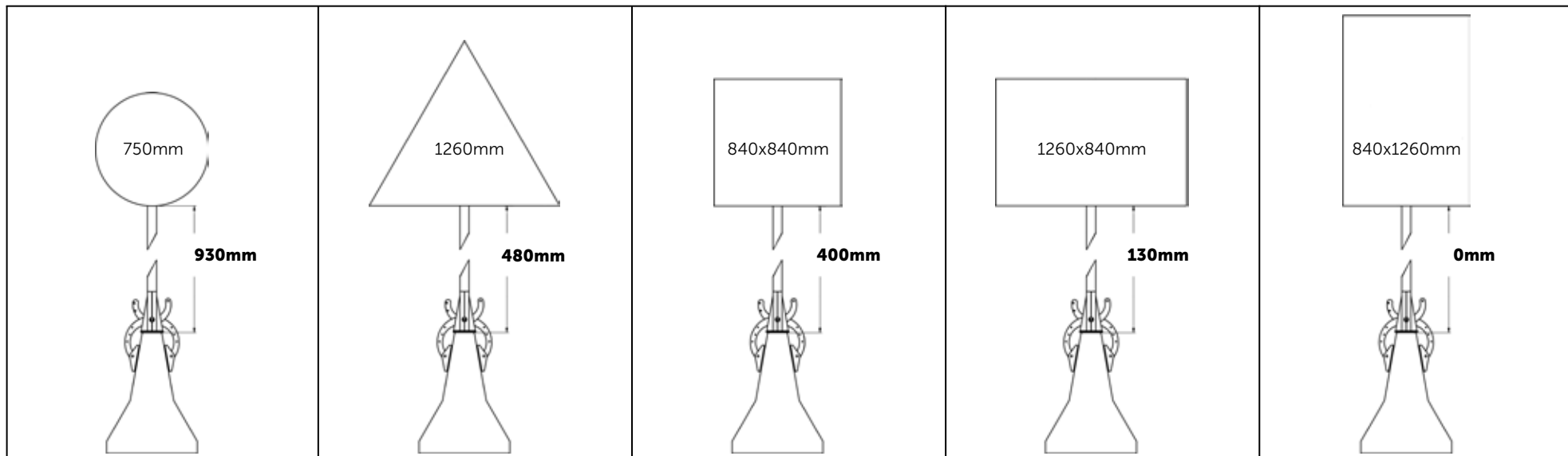
Hauteurs de montage pour panneaux de signalisation taille 3 dans le cas d'une charge de vent de 0,42\text{kn/m}^2 avec 2 TWONG
